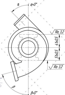
Схема разбора корпуса Вид со стороны турбины
